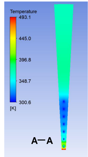
A-A
