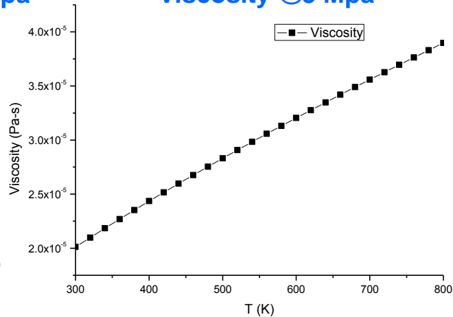
Viscosity @3 Mpa
